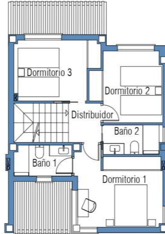
Planta Primera Vivienda 1
